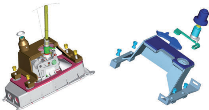
Schematische weergave van de techniek van het slot
